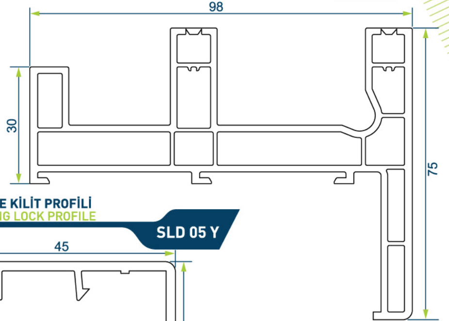
SÜRME SİNEKLİK Lİ KASA PROFİLİ SLIDING FLYING FRAME PROFILE
