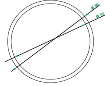
ÜÇ CAM ÇITASI (24 mm) THREE GLAZING BEAD (24 mm)
