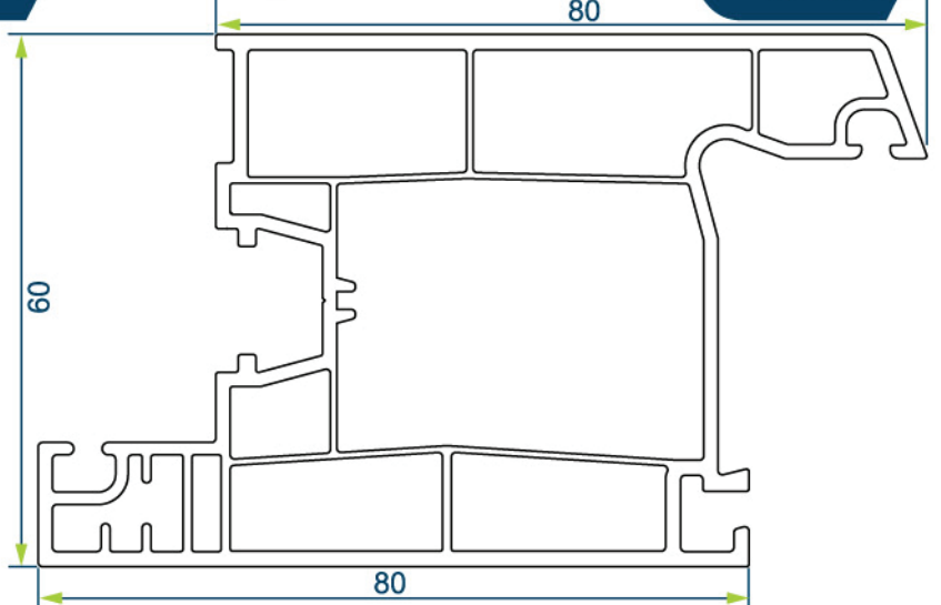
60 mm KAPI KANAT PROFİLİ 60 mm DOOR SASH PROFILE
