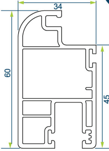
SÜRME KANAT PROFİLİ SLIDING SASH PROFILE
