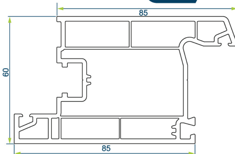
60 mm KAPI KANAT PROFİLİ 60 mm DOOR SASH PROFILE
