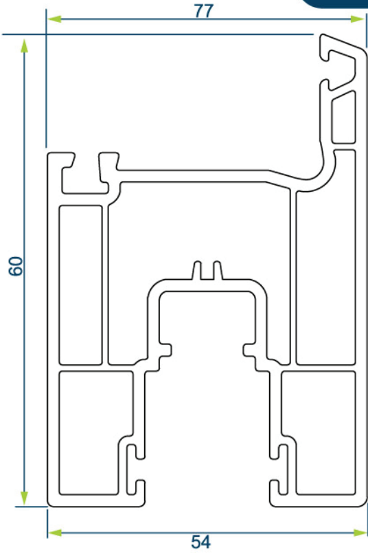
SÜRME KANAT PROFİLİ SLIDING SASH PROFILE
