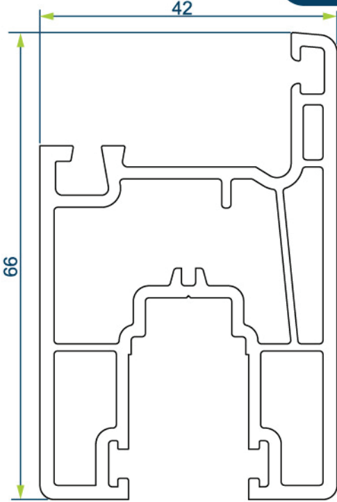
SÜRME KANAT PROFİLİ SLIDING SASH PROFILE
