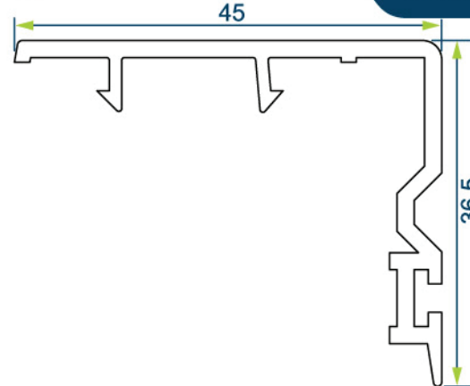
SÜRME KİLİT PROFİLİ SLIDING LOCK PROFILE
