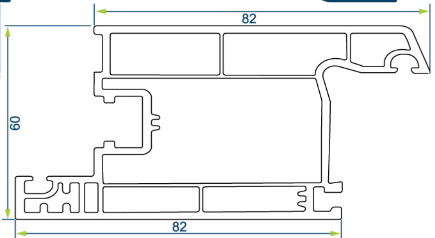
60 mm KAPI KANAT PROFİLİ 60 mm DOOR SASH PROFILE
