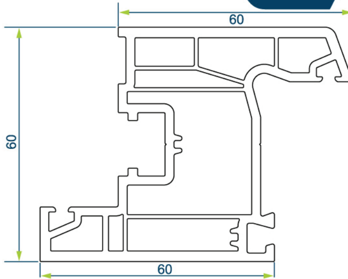
60 mm KAPI KANAT PROFİLİ 60 mm DOOR SASH PROFILE
