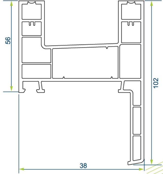
SÜRME SİNEKLİKLI KASA PROFİLİ SLIDING FLYING FRAME PROFILE
