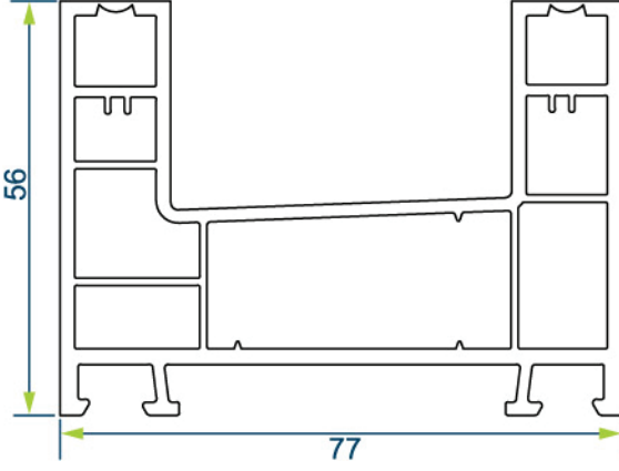
SÜRME KANAT PROFİLİ SLIDING SASH PROFILE
