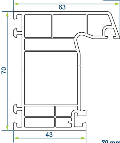
70 mm KASA PROFİLİ 70 mm KASA PROFİLİ
