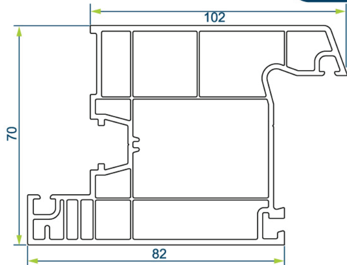
70 mm KAPI KANAT PROFİLİ 70 mm DOOR SASH PROFILE
